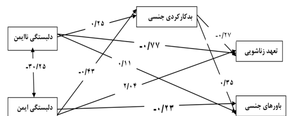
نمودار ۲) ضرایب مسیر مدل پیشنهادی
