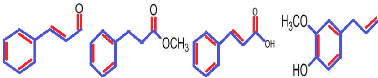
A: Cinnamaldehyde
